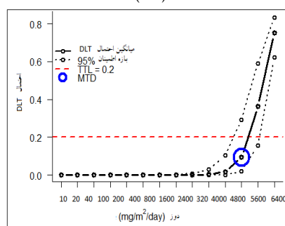
شکل ۶ - نتایج آزمایش دوز یابی در بیماران مبتلا به تومورهای جامد [۲۶] (الف) انجام آزمایش و DLT مشاهده شده (ب) میانگین نهایی برآورد احتمال‌های DLT و بازه اطمینان ۹۵ درصد.
