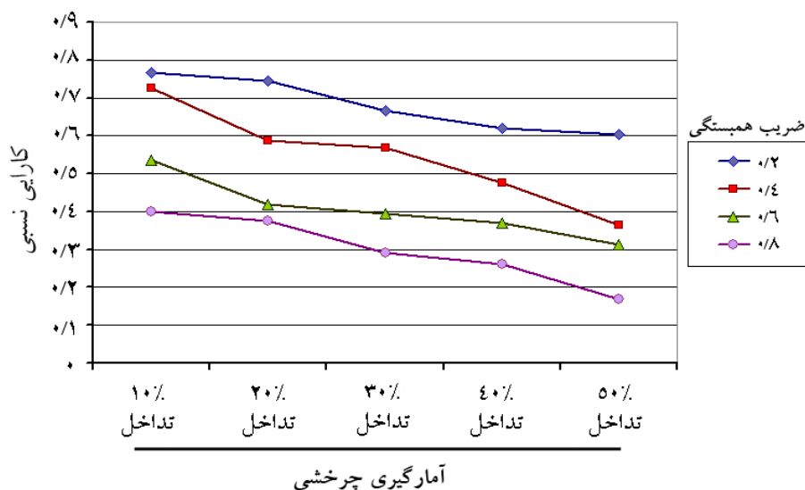
شکل ۱- مقایسه‌ی کارایی برآورد تفاضل میانگین دو دوره با استفاده از رابطه‌ی (۱۸) و تفاضل میانگین نمونه‌ای با در نظر گرفتن ضریب‌های همبستگی مختلف.
